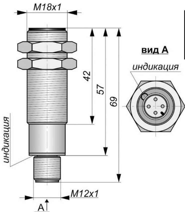
Габаритный чертеж
