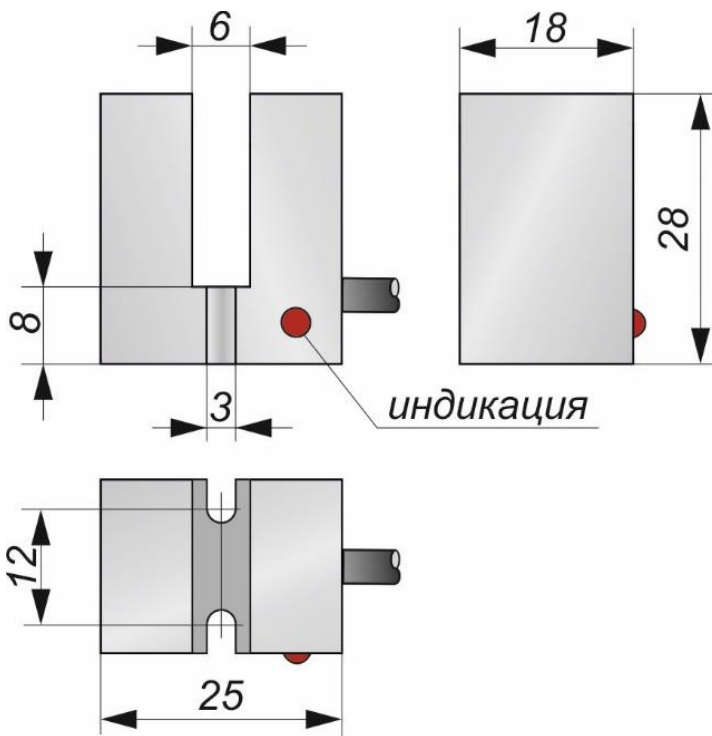
Габаритный чертеж
