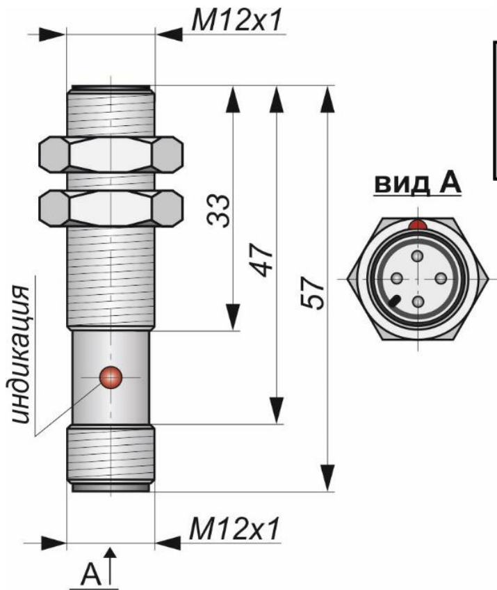
Габаритный чертеж
