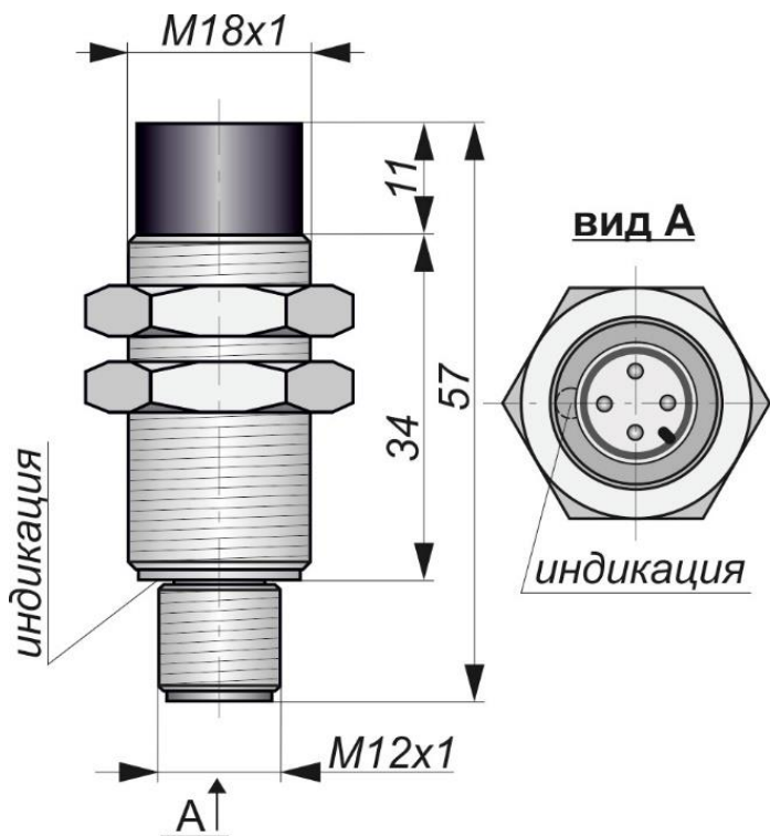
Габаритный чертеж
