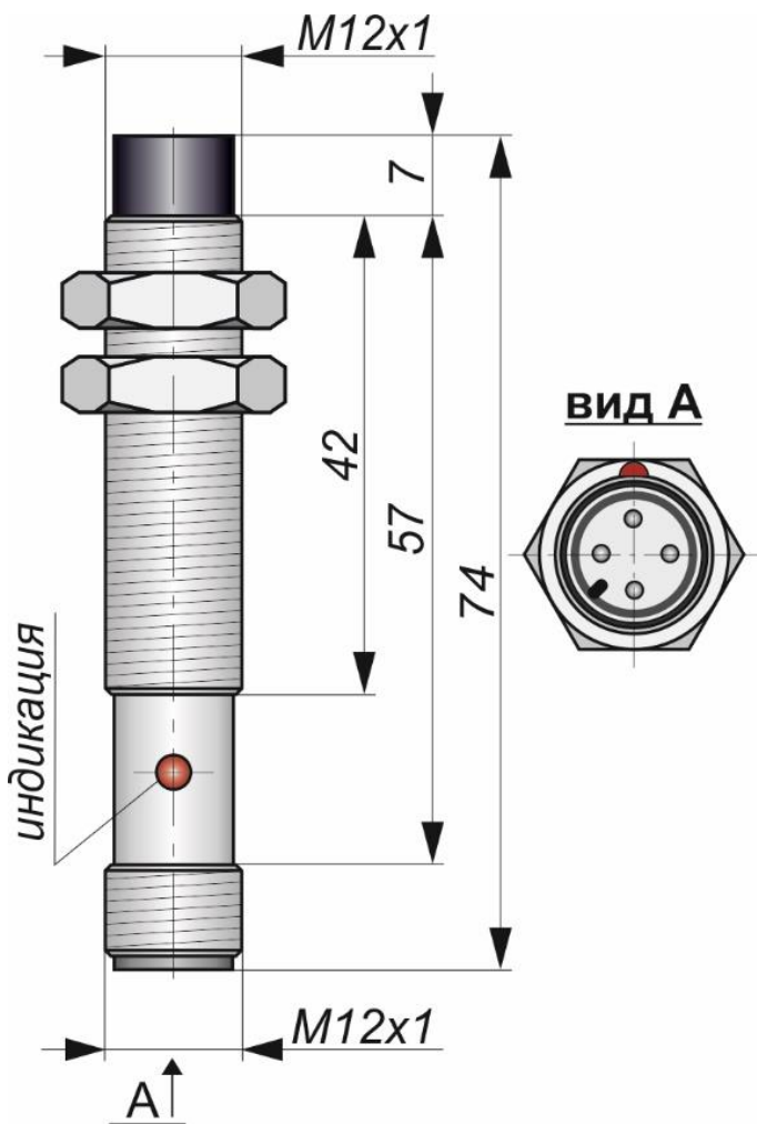
Габаритный чертеж
