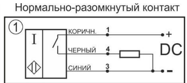
Схема соединения
