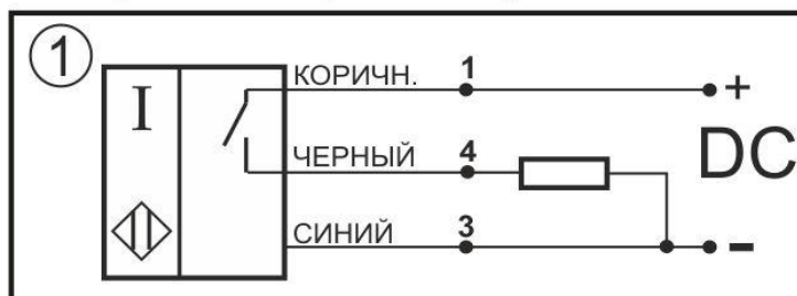
Нормально-разомкнутый контакт
