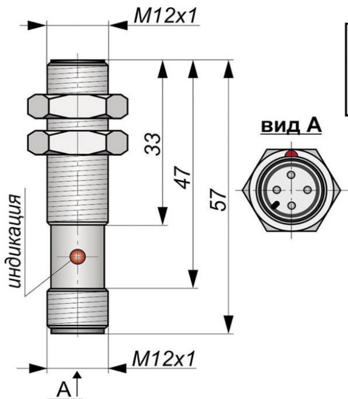
Габаритный чертеж
