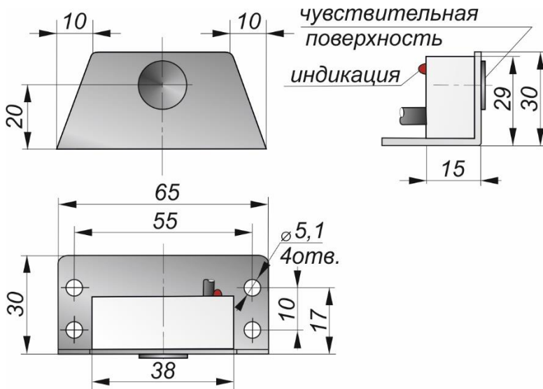
Габаритный чертеж
