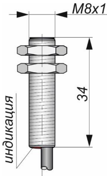
Габаритный чертеж
