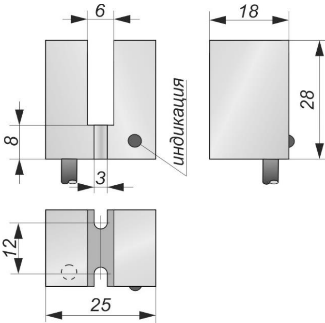
Габаритный чертеж
