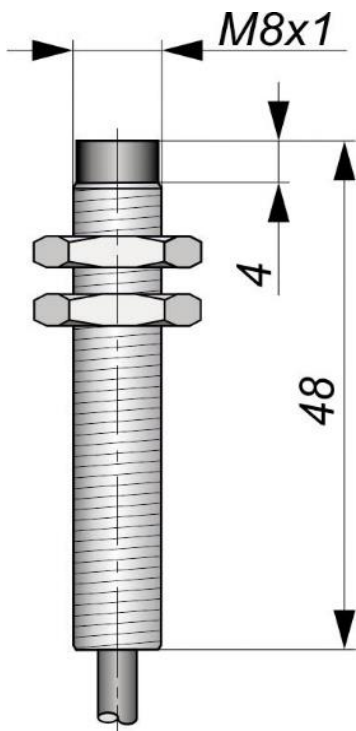
Габаритный чертеж
